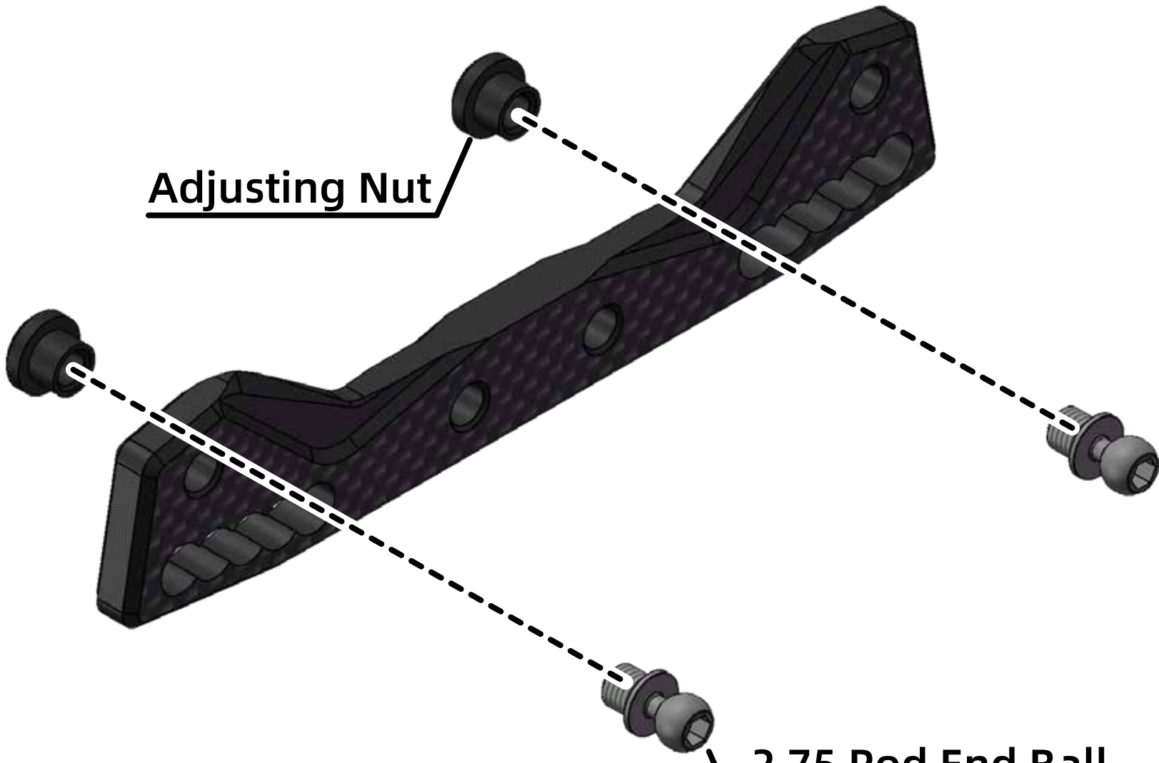
2.75 Rod End Ball
